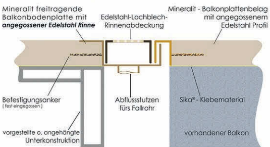
Querschnitt: Entwässerungsbeispiellösung für Mineralit - Balkonbodenplatten
