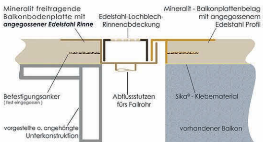
Querschnitt: Entwässerungsbeispiellösung für Mineralit - Balkonbodenplatten
